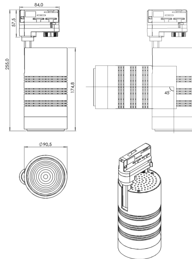
Рисунок 1 Светильник «L-spot 10», «L-spot 20», «L-spot 30», «L-spot 40»
